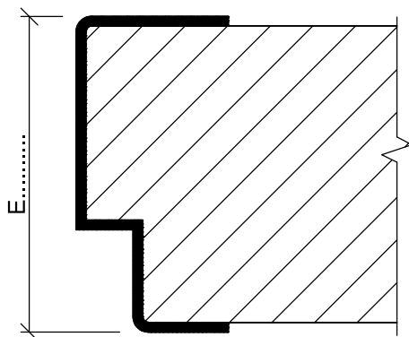
Řez A-A
